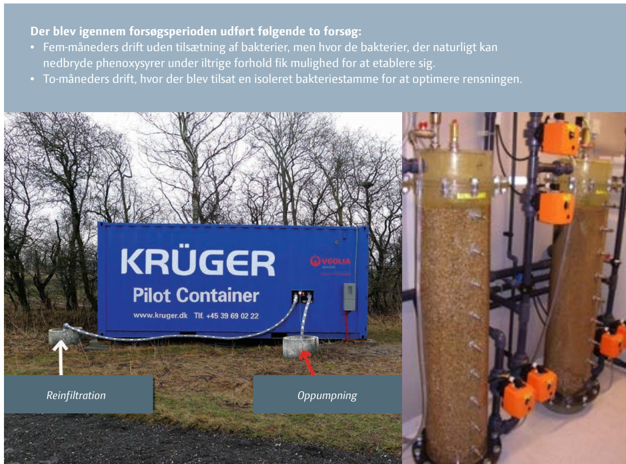
FIGUR 3 - FORSØGSCONTAINER VED BORING 206.1134 OG DE TO BIOLOGISK AKTIVE FORSØGS-SANDFILTRE (30 CM I DIAMETER).
