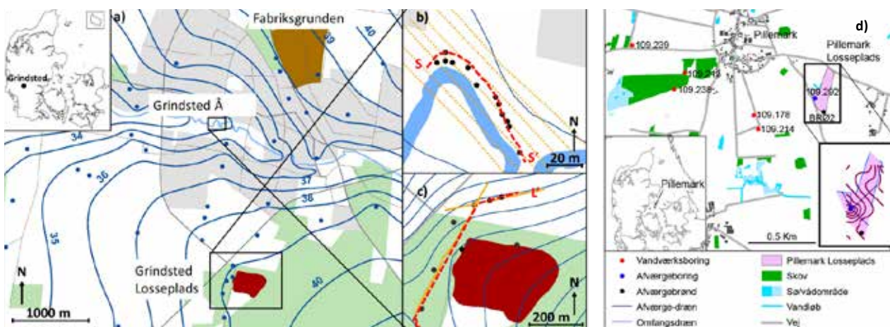
FIGUR 1 OVERSIGTSKORT OVER OMRÅDET VED GRINDSTED MED FABRIKSGRUNDEN, UNDERSØGELSESMÅRÅDET VED GRINDSTED Å OG GRINDSTED LOSSEPLADS SAMT OMRÅDET VED PILEMARK LOSSEPLADS, SAMSØ /1/.
