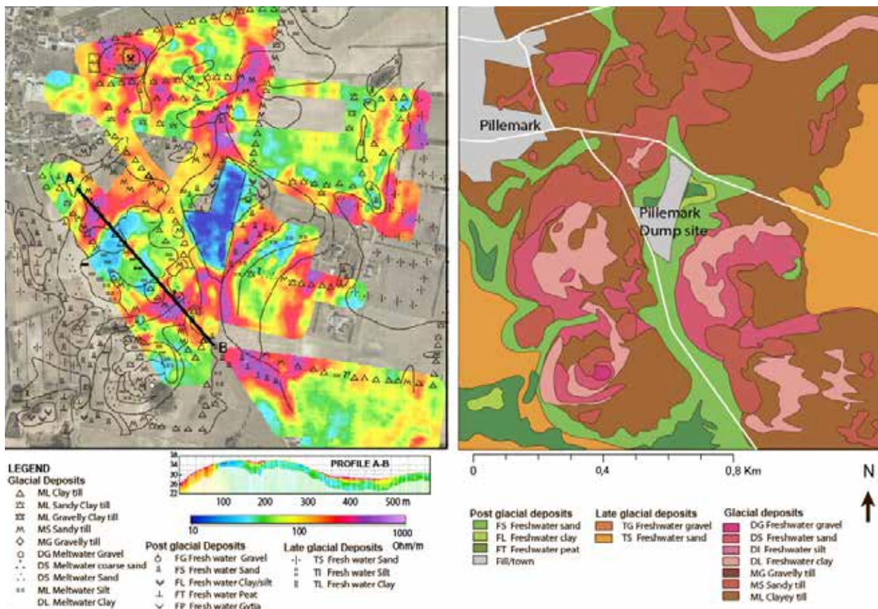
FIGUR 3 DETALJERET GEOLOGISK KORT FOR OMRÅDET OMKRING PILLEMARK LOSSEPLADS PÅ SAMØ UDARBEJDET MED BAGGRUND I DATA FRA GCM MÅLINGER OG OMFATTENDE JORDARTSKARTERING.
