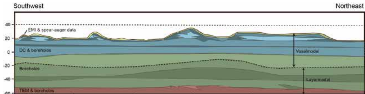
FIGUR 4 EKSEMPEL PÅ OPSTILLING AF EN KOMBINERET LAG- OG VOXEL 3D-MODEL FOR GEOLOGIEN VED LOKALITETEN PÅ SAMØ.
