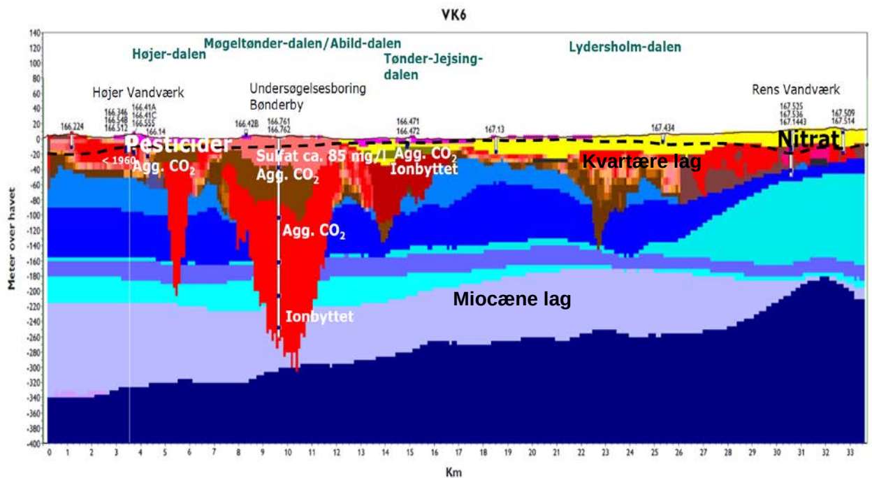
Figur 7.9 Eksempel på principskitse fra grundvandskortlægning ved Tønder (Hansen m.fl., 2015). Stiplet sort linje er dybeste redoxgrænse.
