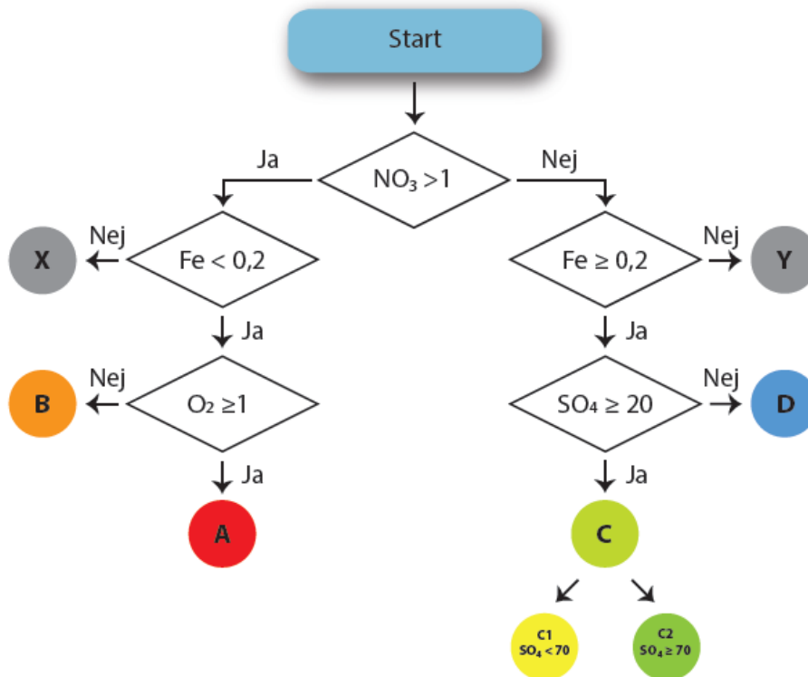
Figur 4.2 Algoritme til fastlæggelse af vandtyper ud fra redoxfølsomme parametre i vandanalyserne.
