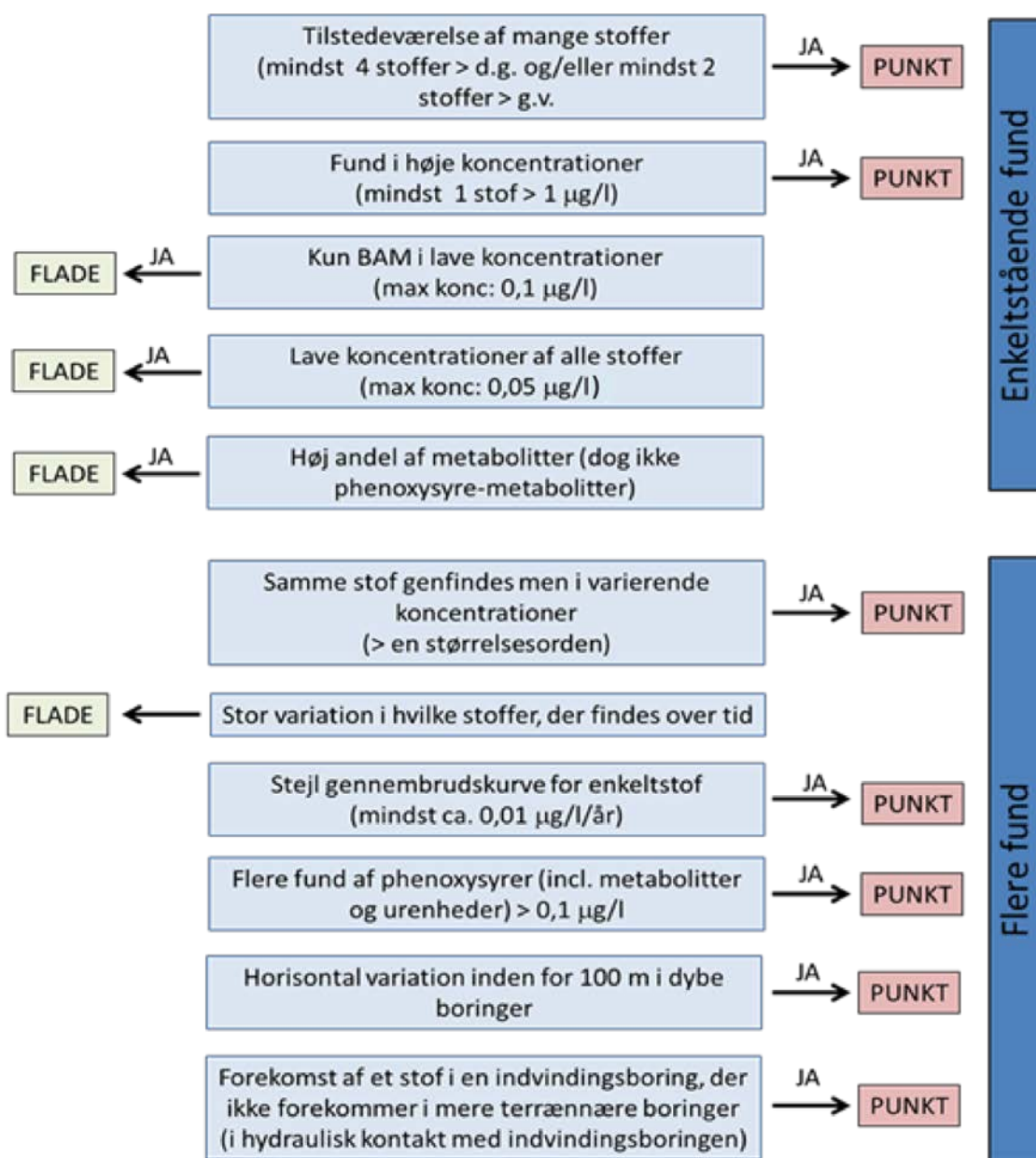
Figur 9.4 Beslutningsstøtte-værktøj til at vurdere kildetypen for pesticidfund i grundvandet (Tuxen m.fl., 2013).
