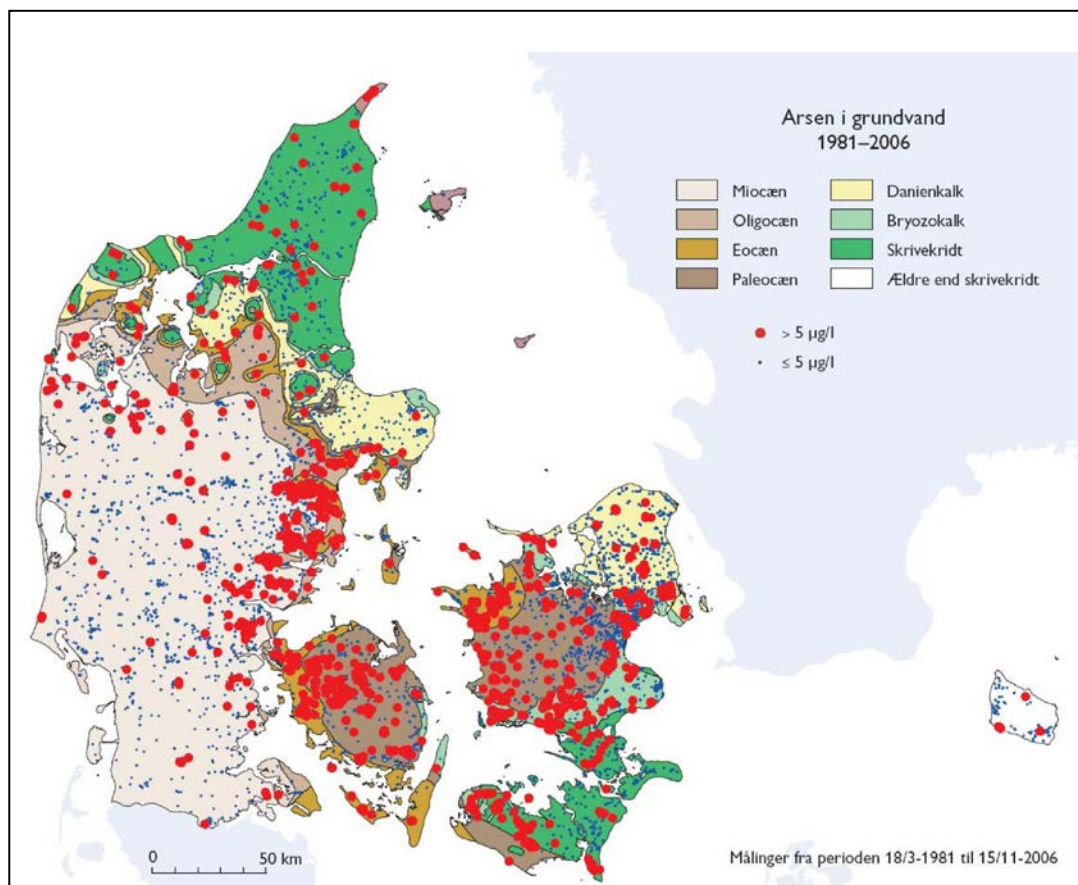
Figur 10.6 Indholdet af arsen i grundvandet i Danmark i forhold til udbredelsen af prækvarter formationer. Analyserne stammer fra forskellige typer borer: LOOP, GRUMO, indvindingsboringer og undersøgelsesboringer (Thorling m. fl., 2007).
