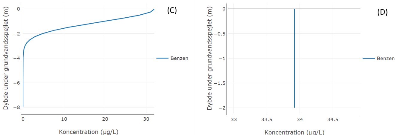
Figur 8.3 (A) Koncentration i kontrolpunktet som funktion af dybden under grundvandsspejlet. B) Eksempel med infiltration over fanen. C) Eksempel uden infiltration over fanen. D) Eksempel for et grundvandsmagasin med mægtighed på 2 m. Her antager modellen, at der er fuld opblanding over dybden og dermed konstant koncentration over dybden.
