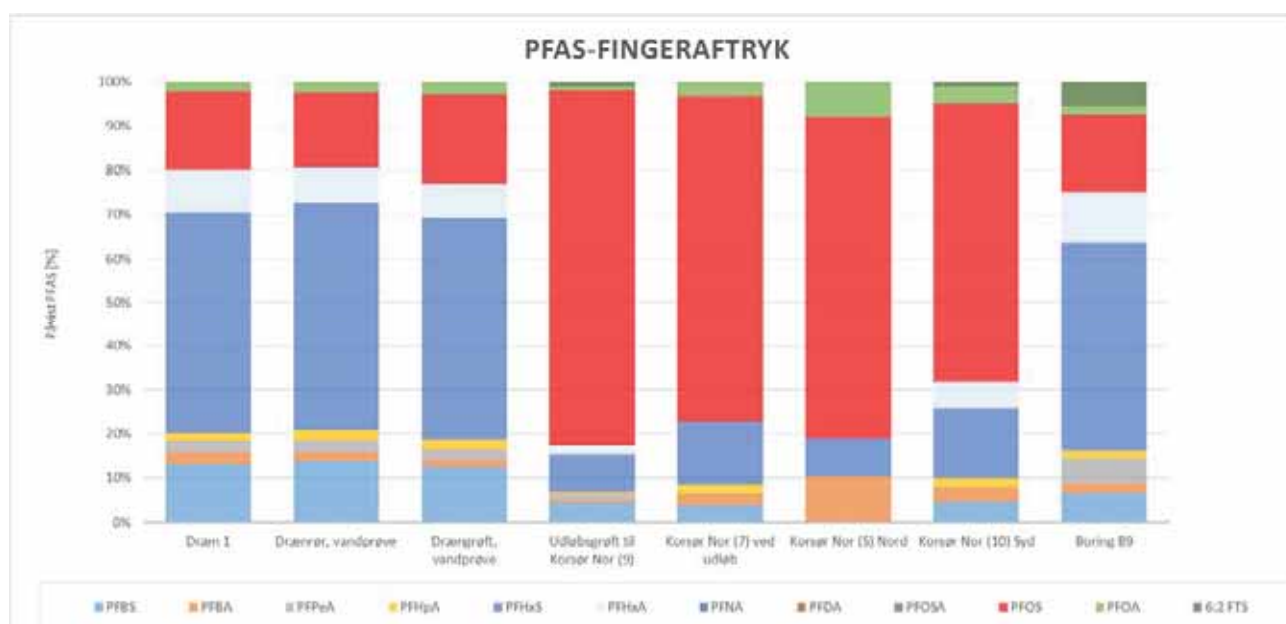
Figur 7.2: PFAS-fingerprint for PFAS påvist i overfladevand.
